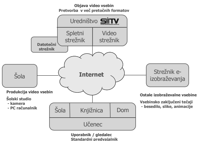
Slika 2: Tehnološka shema
